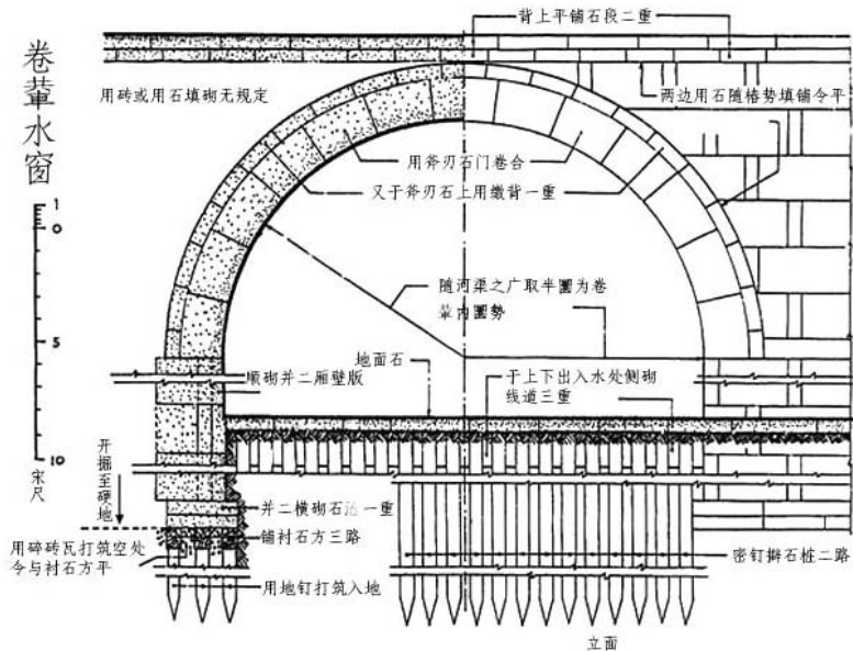
图五 梁思成《营造法式注释》卷上之卷辇水窗图样
