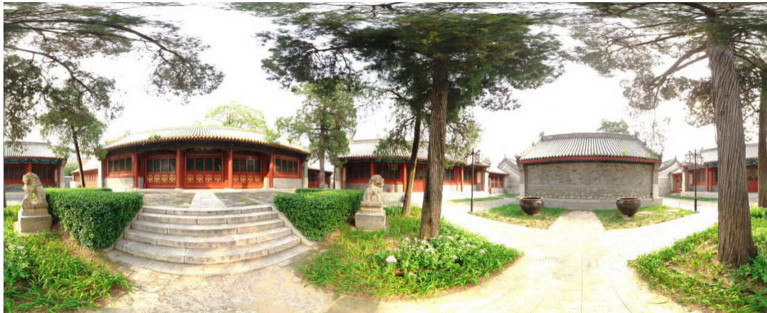
图三 元圣宫地面激光雷达扫描图片
