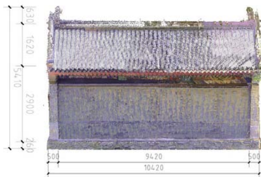
图七 元圣宫前殿背立面图
