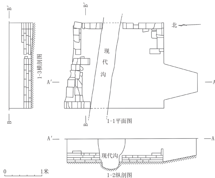
图八 M2平、剖面图
