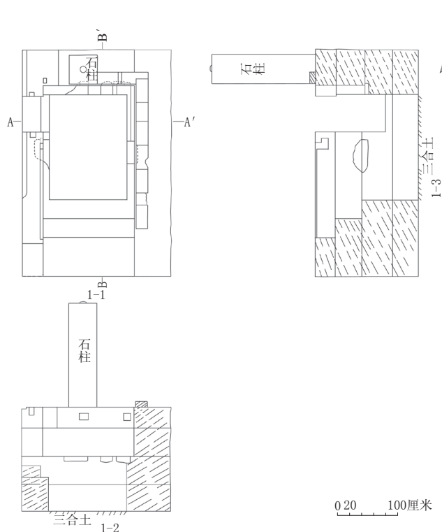
图一四 水车汲水池2平面图及四壁立面图
