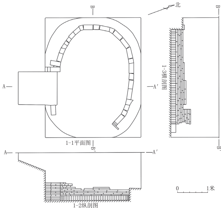
图七 M1平、剖面图
