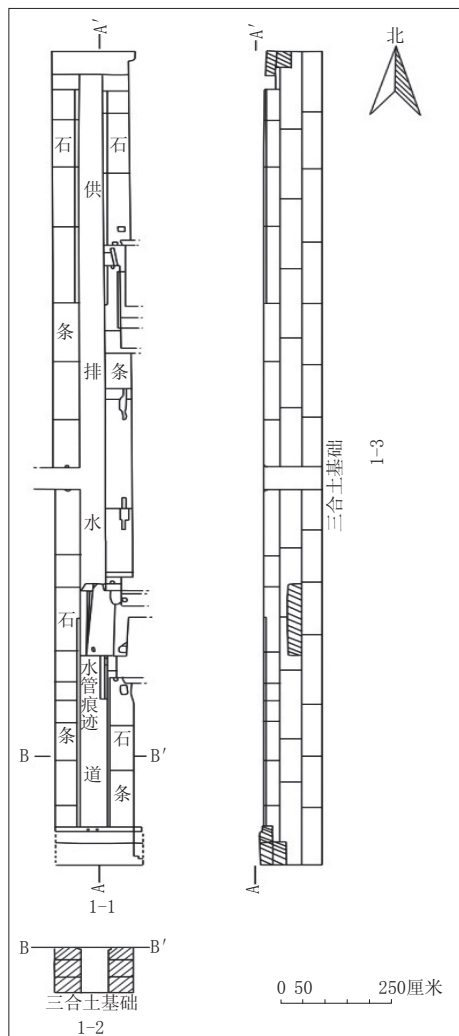
图四 水道1平、剖面图
