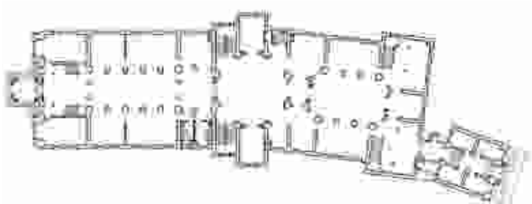
图五 大栅栏劝业场现状首层平面图
